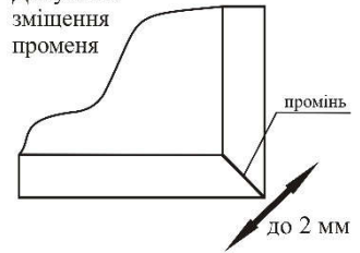
Притуплення кутів
